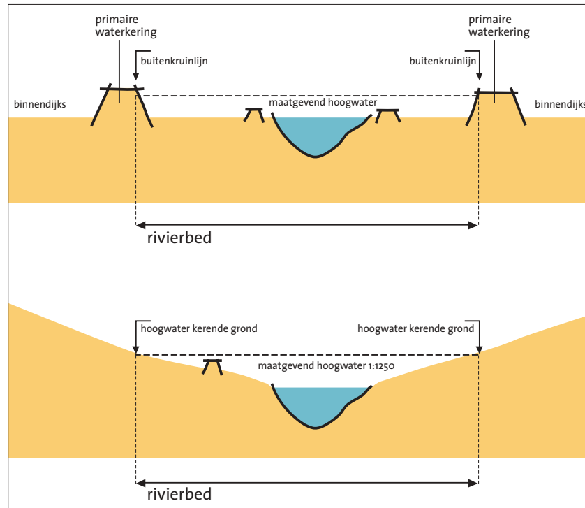
Figuur 1 Een schematische weergave van het rivierbed, als vastgelegd in de Wbr in een bedijkte (boven) en onbedijkte (onder) situatie.
