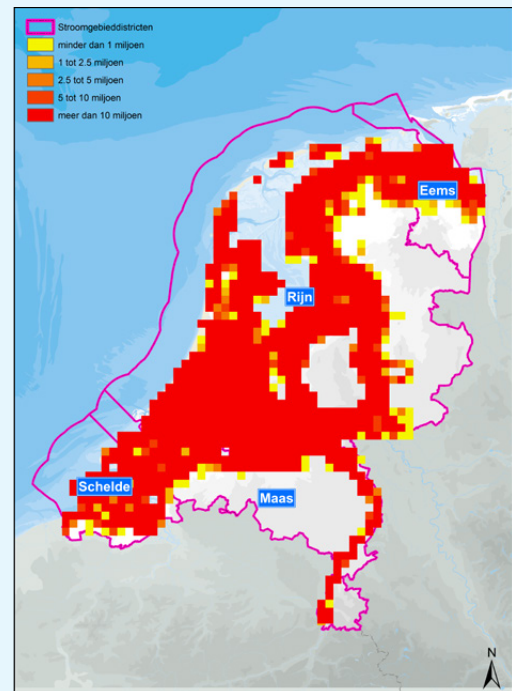
Overstroming als gevolg van doorbraak van een primaire kering langs het hoofdwatersysteem (B)
